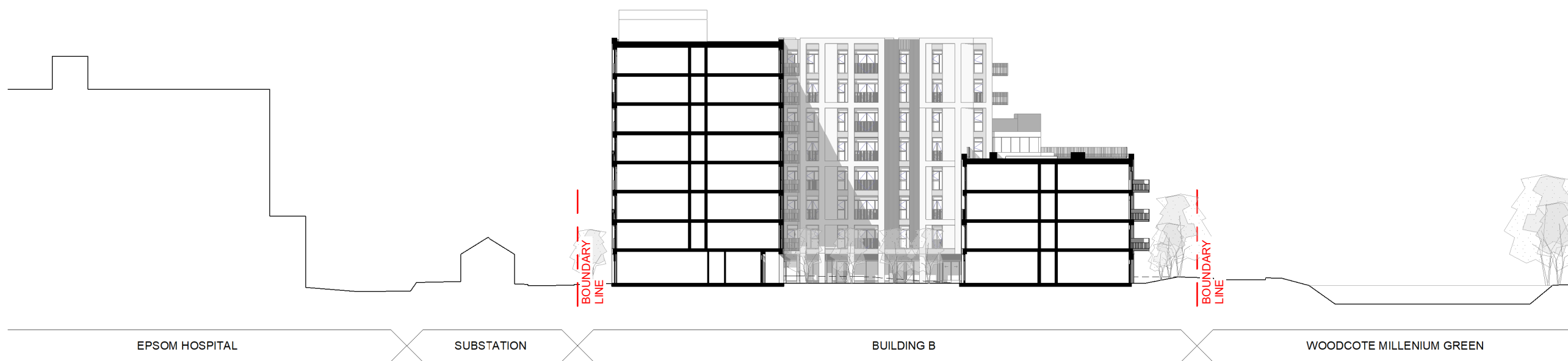
SITE SECTION BB 1 : 500
