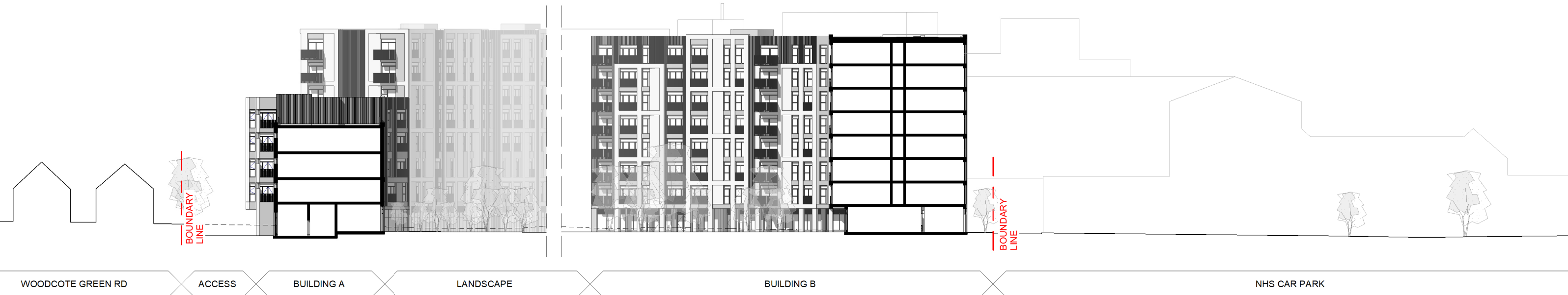
SITE SECTION DD 1 : 500
